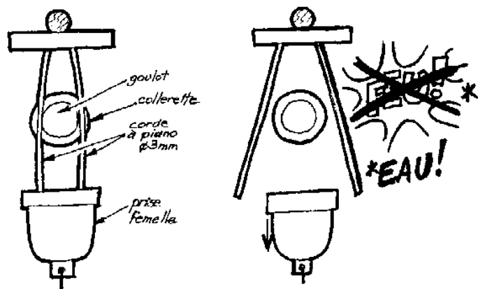
détails du système de déclenchement.
